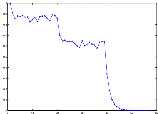
(c) \frac{\|z_s(t) - p_s\|}{\|z_s(0) - p_s\|} w.r.t. t
